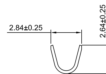
SEC:A-A
