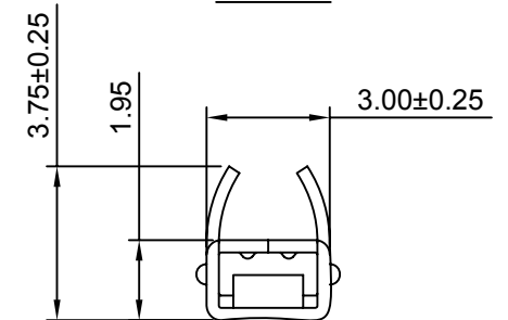
SEC:B-B
