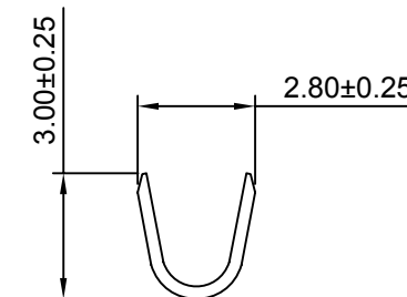
SEC:B-B
