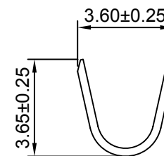
SEC:B-B
