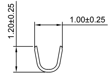
SEC:A-A
